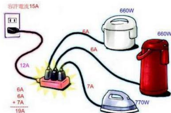
圖 3-12 電流超過負荷
