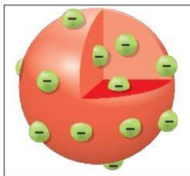
Modelo atômico de Thomson
