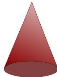
cone
