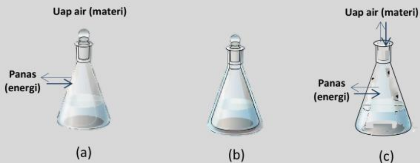
Gambar 2. Jenis sistem termokimia (Jespersen et al. , 2017:260)
