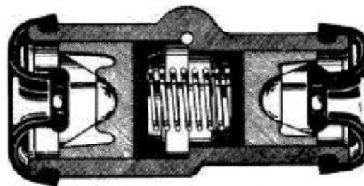
Gambar 1. 13 Silinder roda bertingkat
