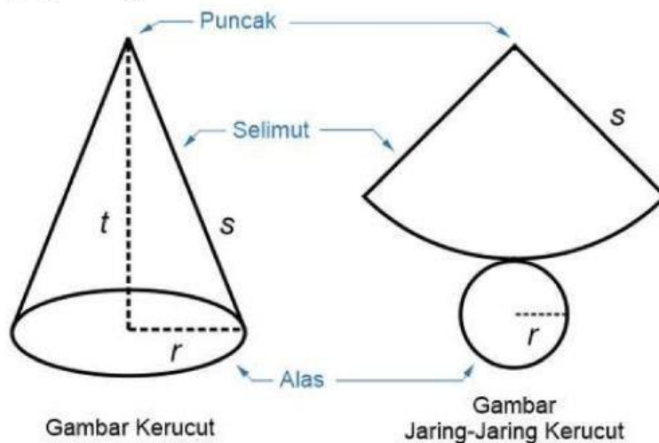
Gambar 1. Jaring-jaring Kerucut
