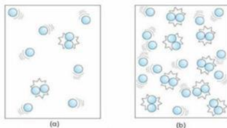
Gambar 2.2 Reaktan dengan konsentrasi yang berbeda Sumber: Lewis, Thinking Chemistry
