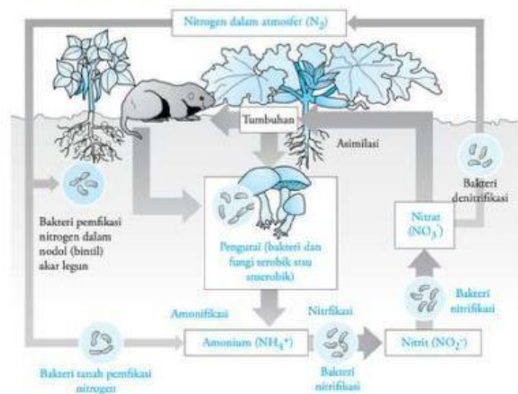
Gambar 15. Siklus Nitrogen
