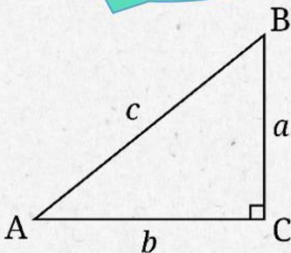
Gambar 1.5 Segitiga Siku-siku
