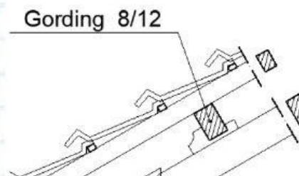
g. Gording
