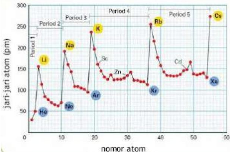
Grafik jari jari atom dan nomor atom
