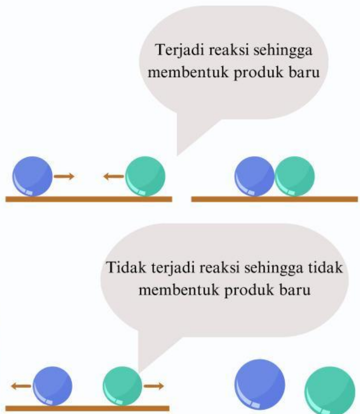
Gambar 2. Tumbukan antar molekul
