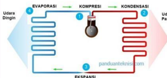
Gambar 3. Prinsip Kerja AC (sumber : Edutech.com)
