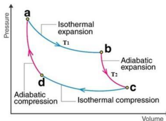
Gambar 2. Siklus Carnot
