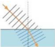
การหักเห
