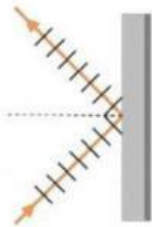
การสะท้อน
