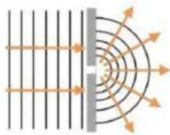
การเลี้ยวเบนของคลื่น
