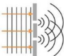
การหักเหของคลื่น
