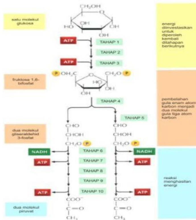
Gambar 4. Tahap Glikolisis
