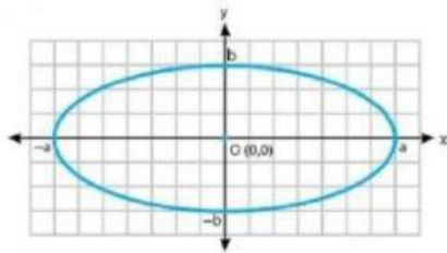
Gambar elips horizontal di pusat O(0,0)
