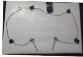
Gambar 4. Rangkaian alat uji daya hantar listrik
