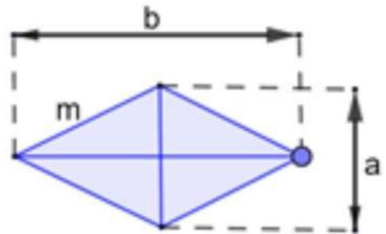
Hình thoi
