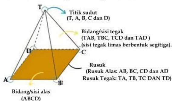
Gambar 8. Unsur-unsur Limas Segiempat
