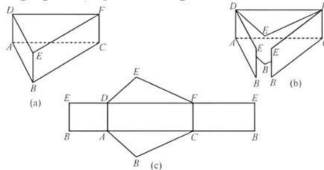
Gambar 7. Jaring-jaring Prisma segitiga
