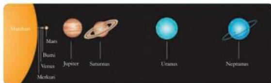
Gambar 7.2 Delapan planet dalam Tata Surya. Sumber: Pearson Heinemann/Wendy Gordon (2009)
