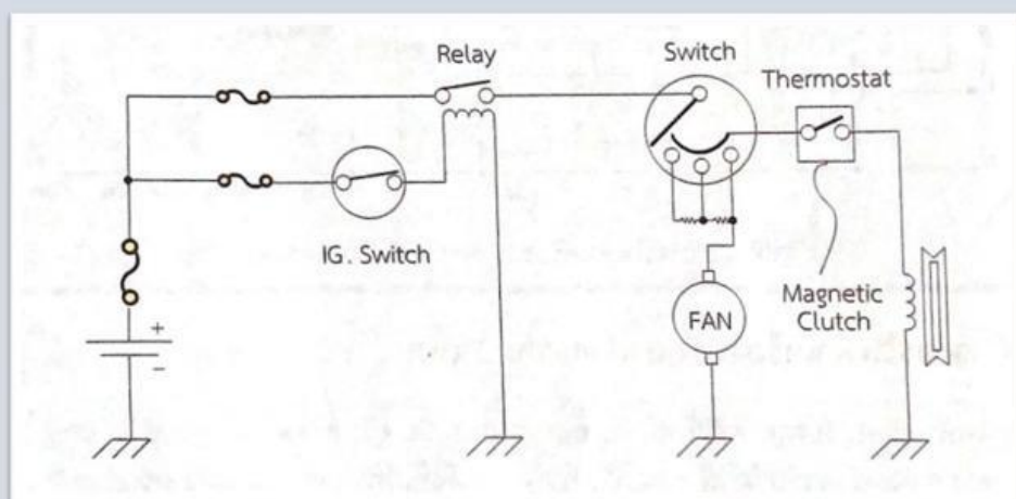
วงจรไฟฟ้าเครื่องปรับอากาศรถยนต์
