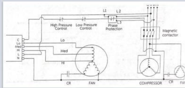
วงจรไฟฟ้าเครื่องปรับอากาศที่ใช้ไฟฟ้า 3 เฟส
