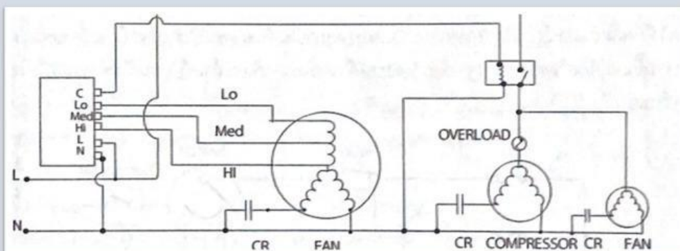
วงจรไฟฟ้าเครื่องปรับอากาศแบบใช้กล่องควบคุม
