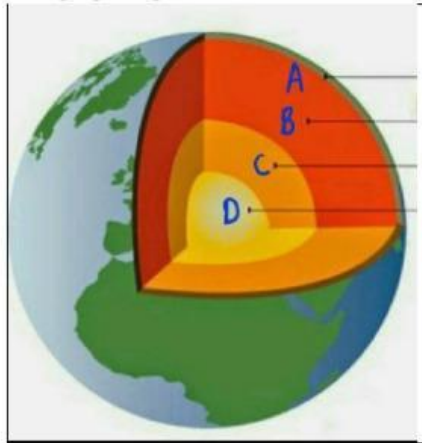
Gambar 1. Lapisan Bumi
