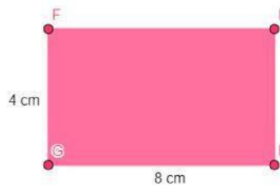
Gambar 8. Persegi panjang BCDE dan Persegi Panjang FIHG
