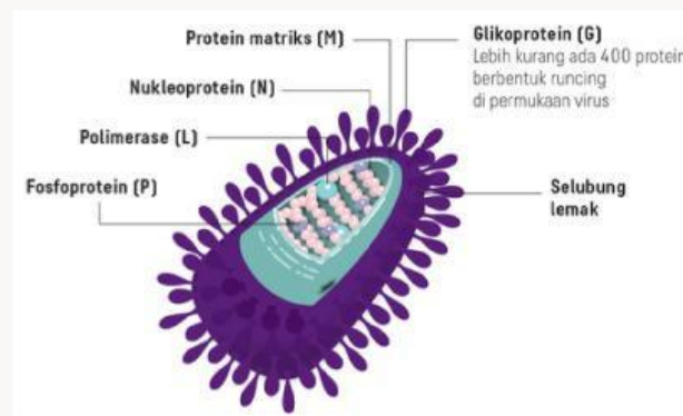
Gambar 1.2 Bentuk Virus
