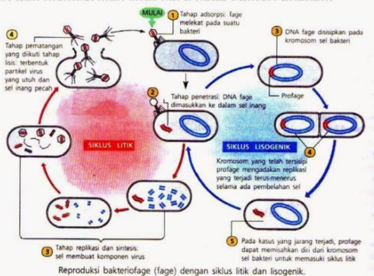
Gambar 1.6 Reproduksi Bakteriofage
