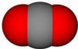
Molekul CO 2
