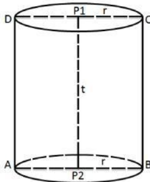
Gambar 2. Bangun Tabung
