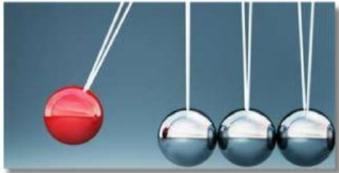
Gambar 2. Animasi Bandul
