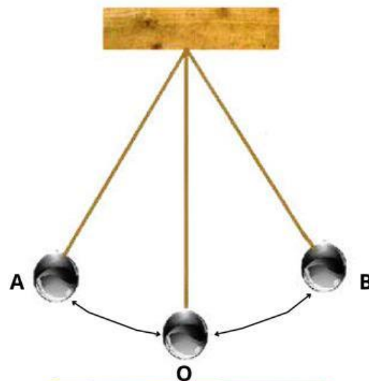
Gambar 1. Simulasi Bandul
