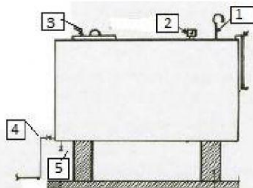
Τυπική δεξαμενή υγρών καυσίμων
