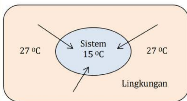
Gambar 3. Contoh kondisi penyerapan kalor (Endoterm)
