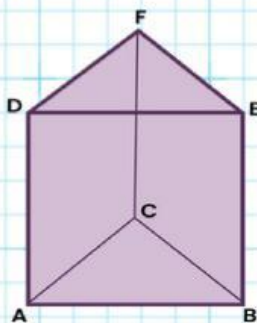
Prisma Segitiga
