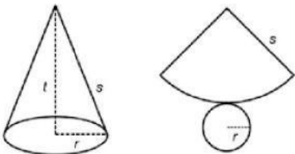
Kerucut
