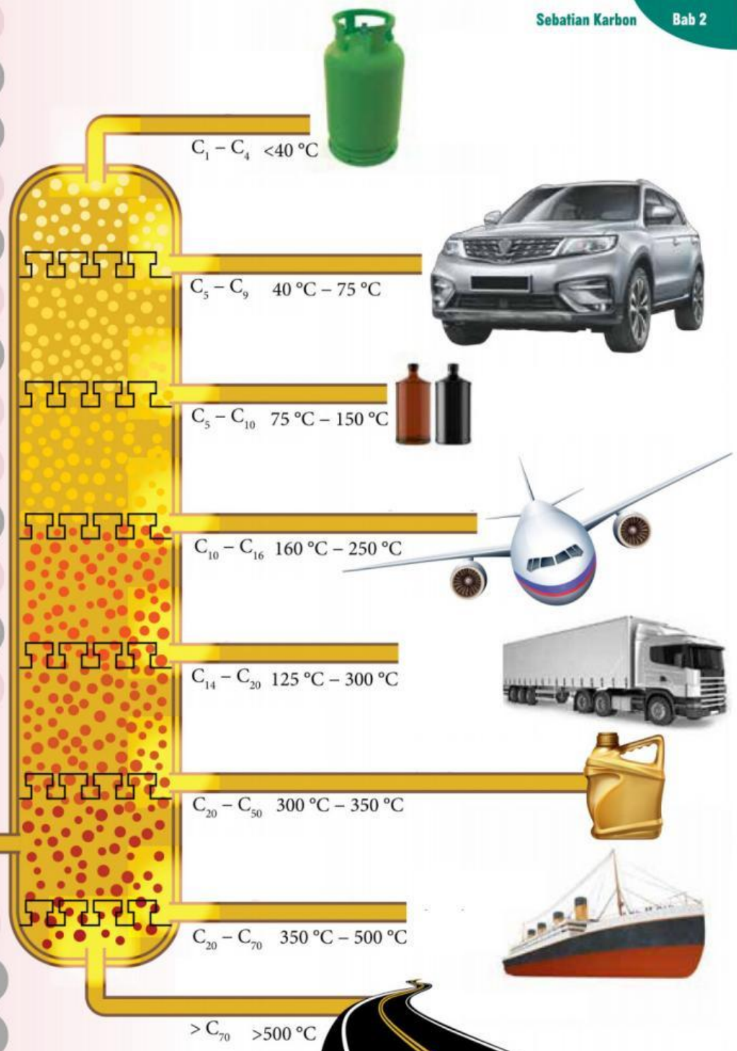
Rajah 2.2 Proses penyulingan berperingkat petroleum dan kegunaan hasilnya dalam kehidupan seharian
