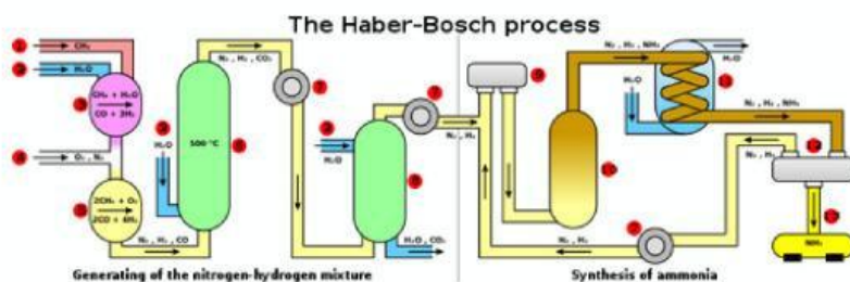
Gambar 1.6. Proses Haber-Bosch
