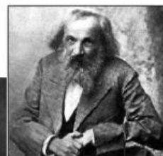
D. Mendelejew
