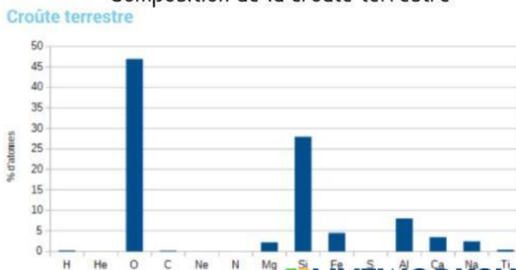
Composition de la croûte terrestre
