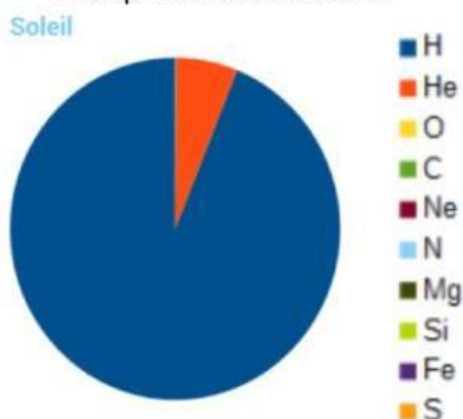
Composition du soleil
