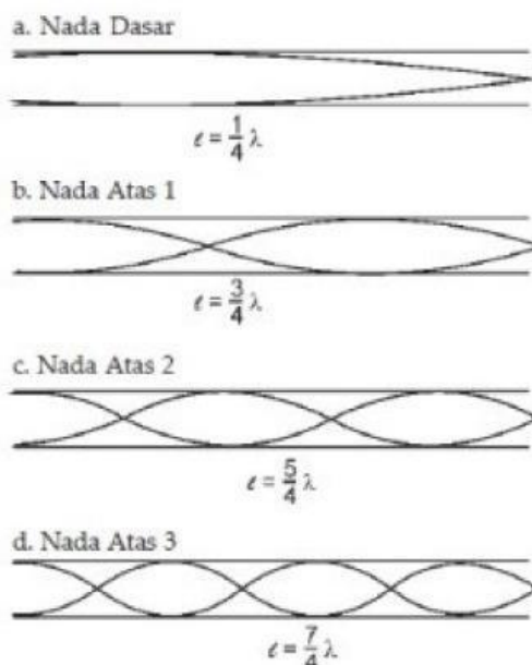
Gambar 1.4 Pola Gelombang Stasioner pada Pipa Organa Tertutup Sumber: Zenius
