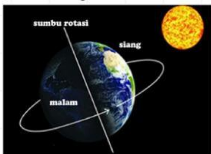
Gambar 22. Gerak Rotasi Bumi
