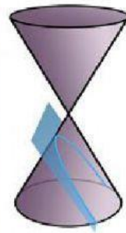
Parábola
