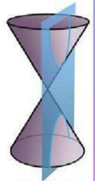
Hipérbola
