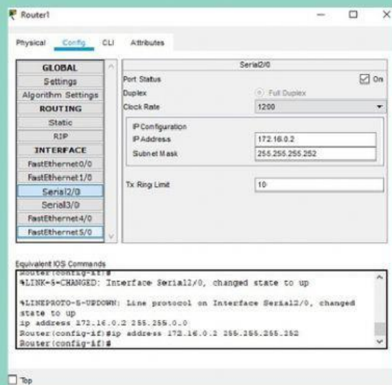
Gambar 9. Konfigurasi Serial Router1
