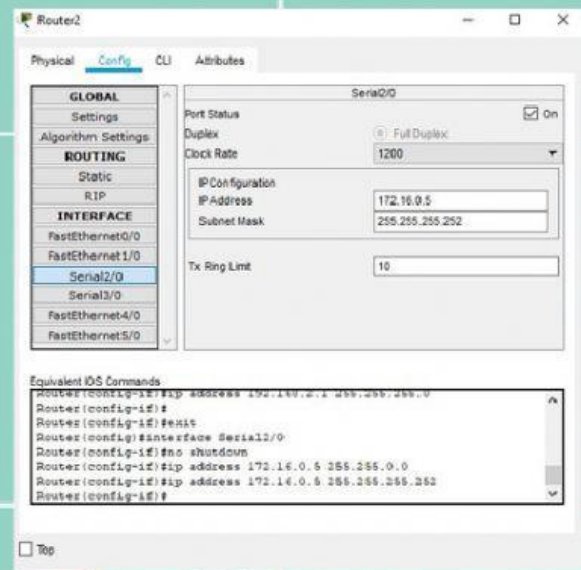
Gambar 34. Konfigurasi Serial Router2
