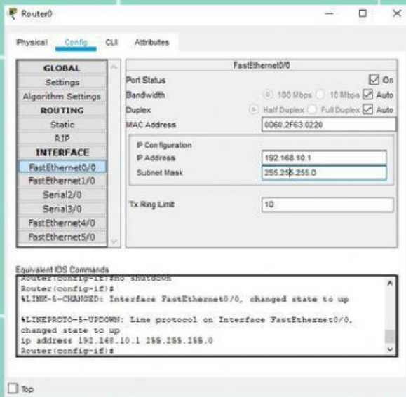
Gambar 31. Konfigurasi FastEthernet Router0
