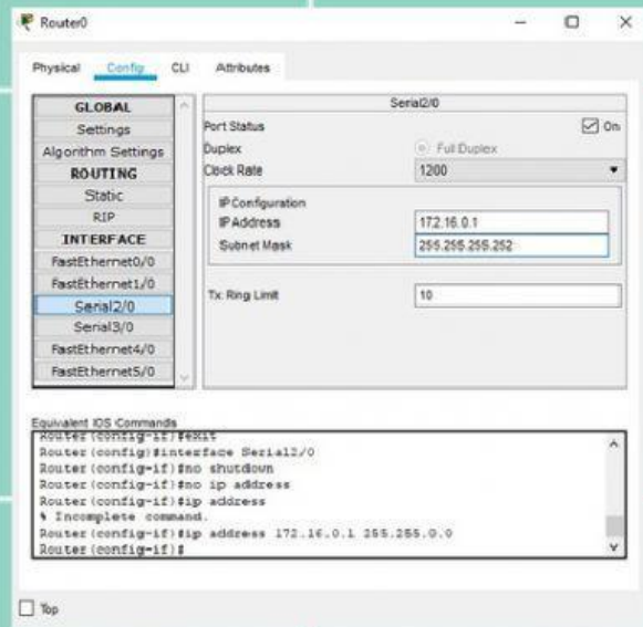
Gambar 32. Konfigurasi Serial Router0
