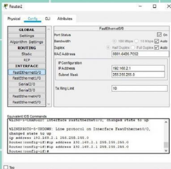
Gambar 33. Konfigurasi FastEthernet Router2
