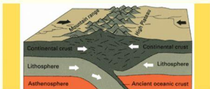
Gambar 4 Pergerakan Lempeng Tektonik (Sumber: ruangguru.com)
