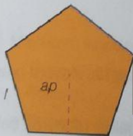
Poligono erregularra
