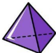
τριγωνική πυραμίδα
