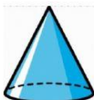
κώνος
