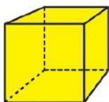
CUBO
