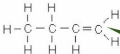
but-1-ene
