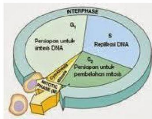
Gambar 4.1 Siklus Sel
