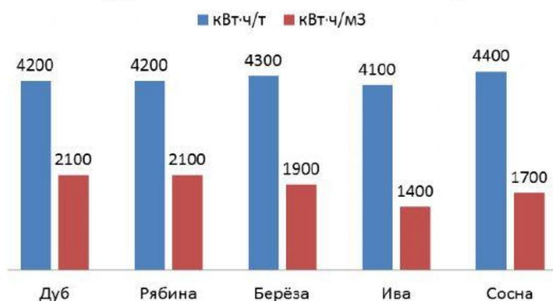
Теплотворная способность видов древесины (удельная теплота сгорания топлива)
