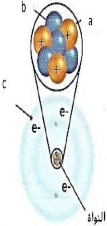
ذرة الليثيوم
