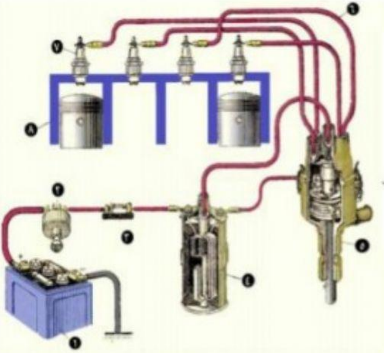
دورة إشعال ببطارية
