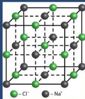
поваренная соль
