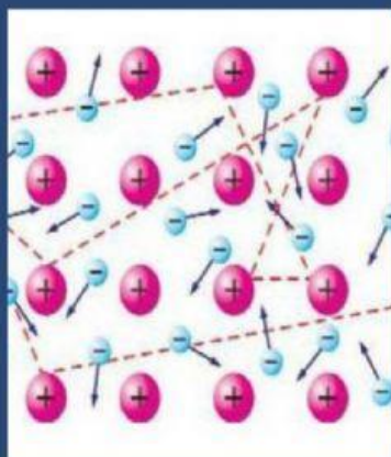
медь
