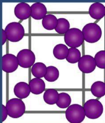
иод
