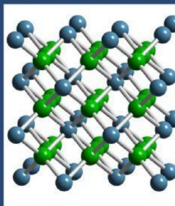
кварц
